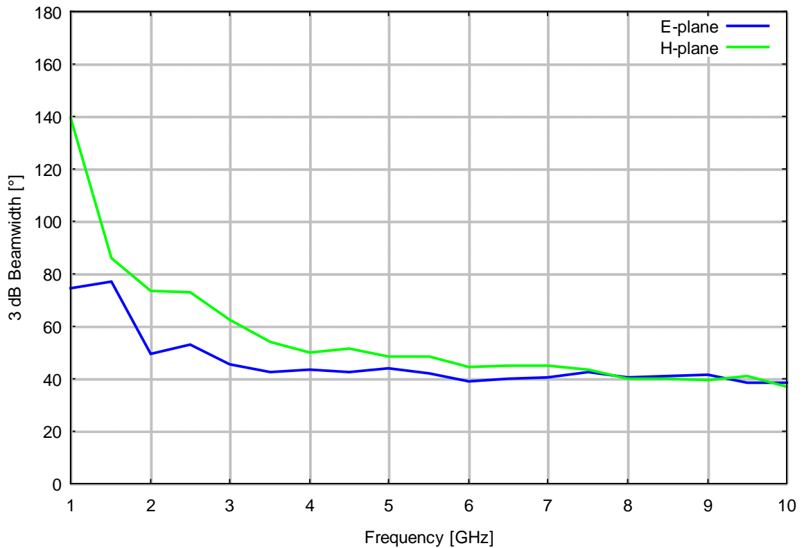
3 dB Öffnungswinkel
