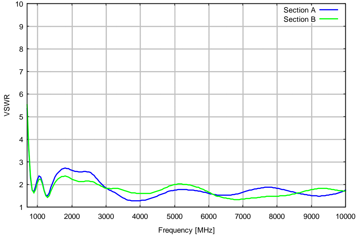
Stehwellenverhältnis
